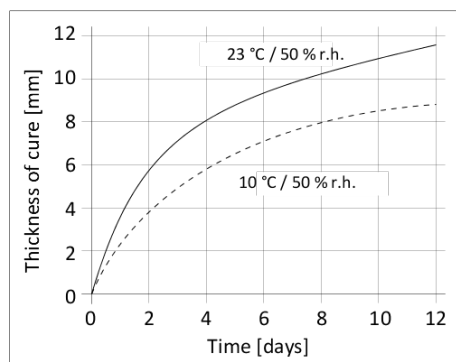
Diagramma 1: Velocità di indurimento per Sikaflex®-290 DC PRO
